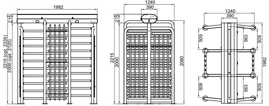
Ölçüler (mm)
