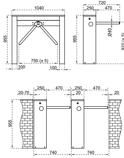
Ölçüler (mm)
