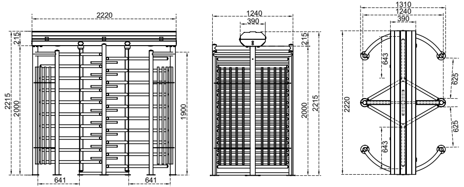
Ölçüler (mm)
