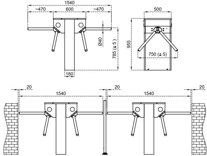
Ölçüler (mm)
